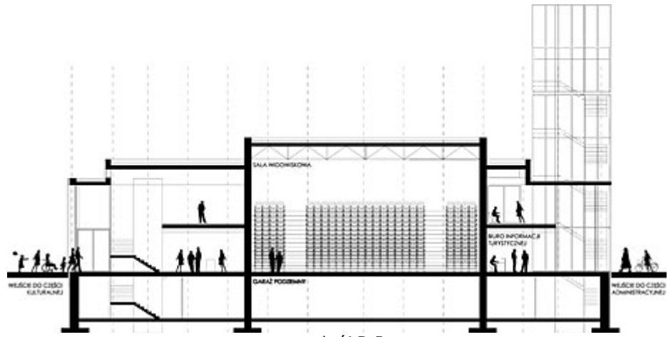
przekrój B-B
