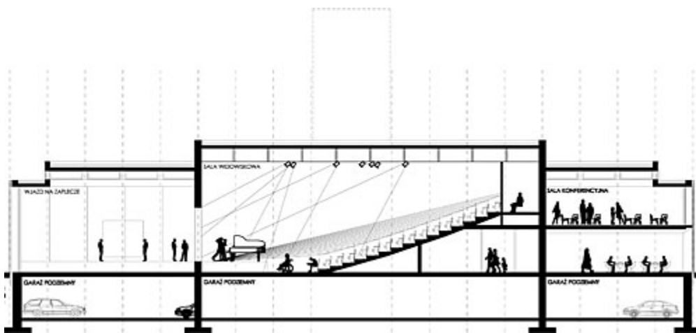
przekrój A-A
