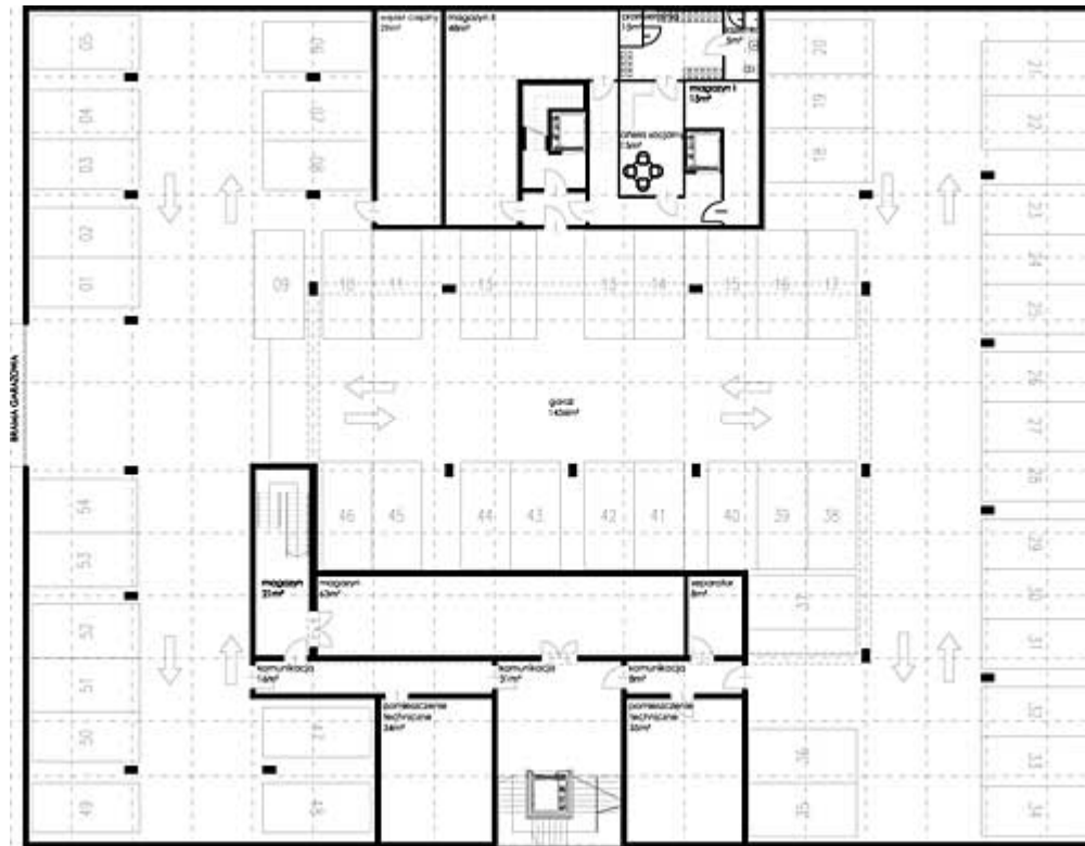
rzut garażu
